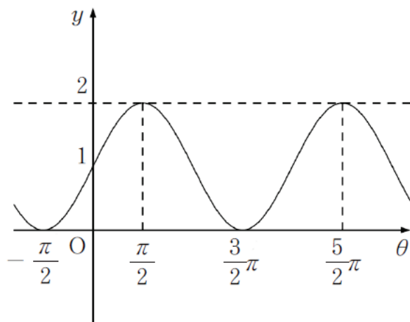
(3) 周期 2\pi
