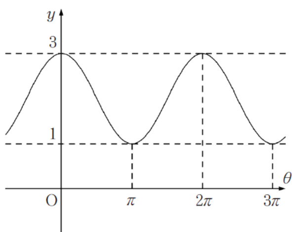
(4) 周期 2\pi
