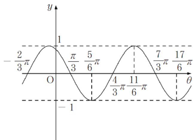
(2) 周期 2\pi
