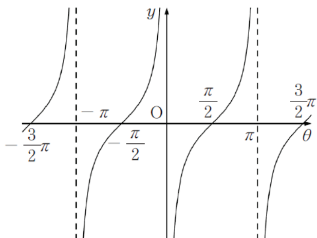
(1) 周期 \pi
